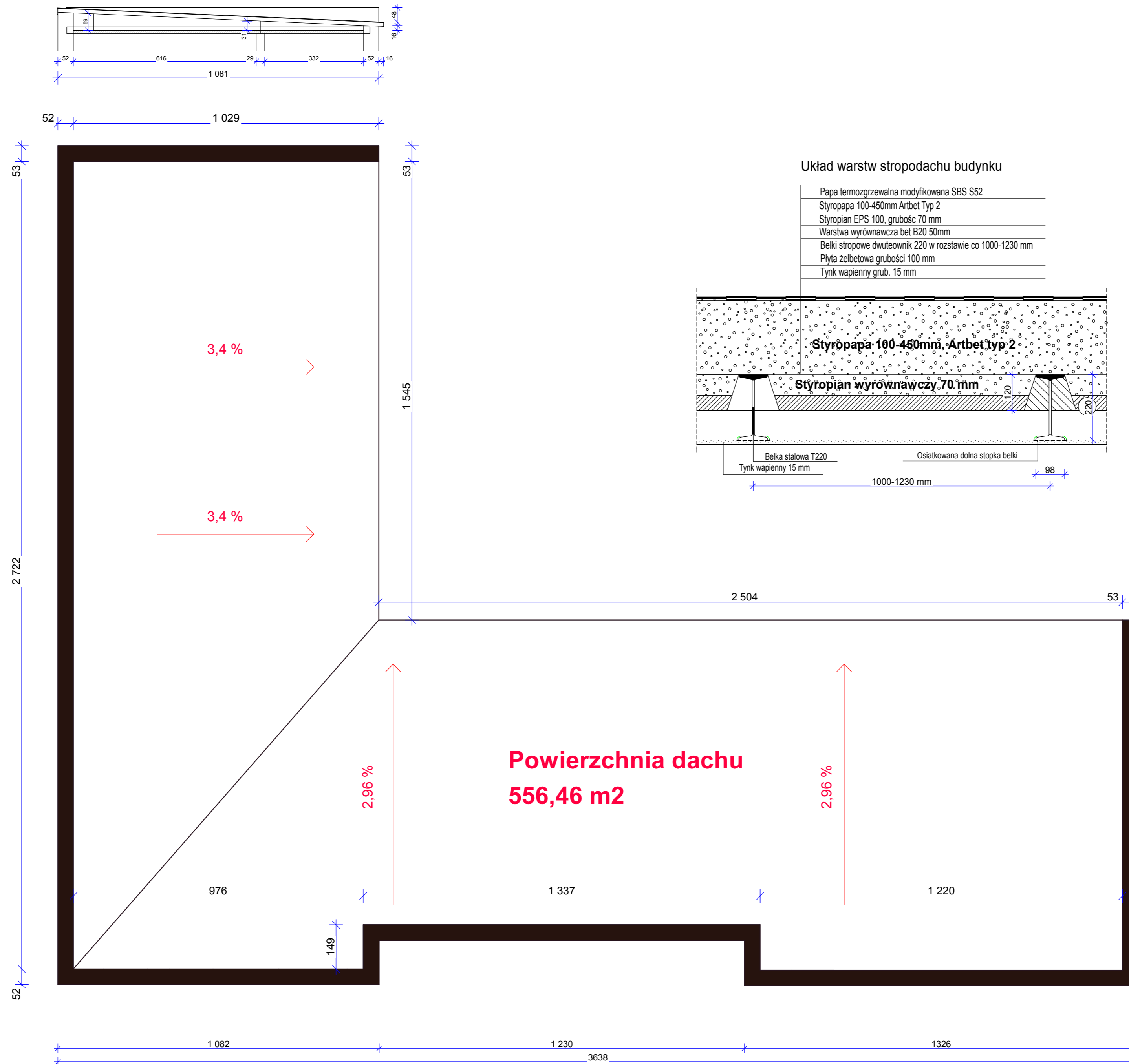
Rys. 5.2. Rzut dachu Szkoły Podstawowej w Charzynie
